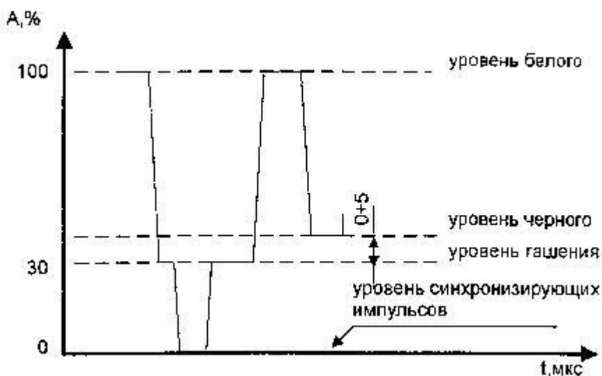
Рисунок П.2.1. Уровни входного видеосигнала
