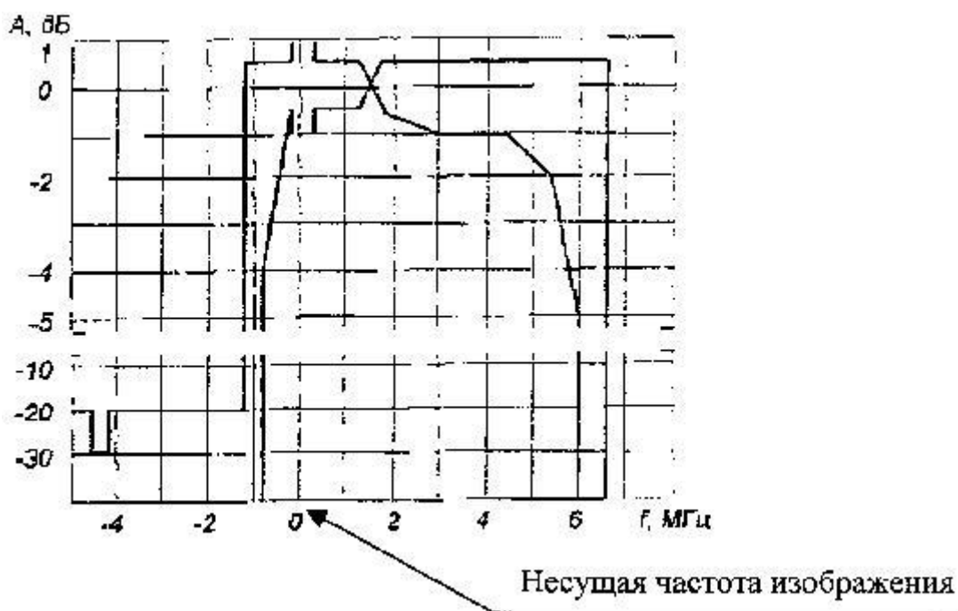
Рисунок П.4.1. АЧХ боковых полос аналогового передатчика
