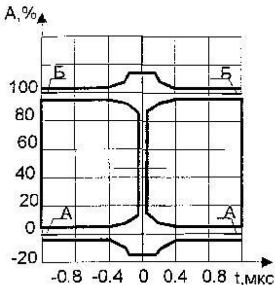
Рисунок П.2.3. Поле допуска переходной характеристики
