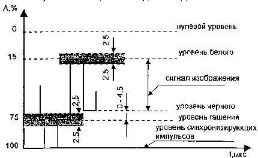
Рисунок П.2.2. Уровни выходного радиосигнала изображения
