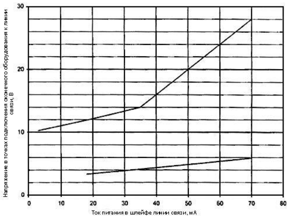
Рисунок П.2.1. Зависимость напряжения в точках подключения к линии связи от тока питания в замкнутом шлейфе линии связи
